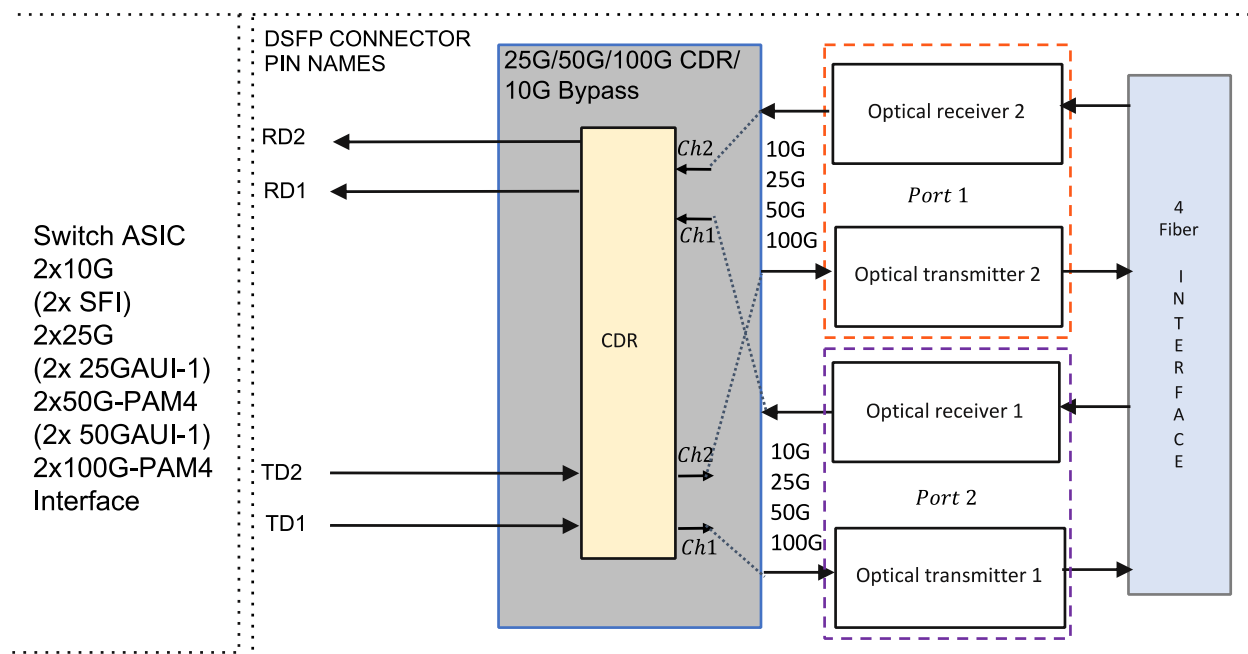
Figure 1: Block diagram for 10/25GBASE-SR/LR or 50GBASE-SR/FR/LR
